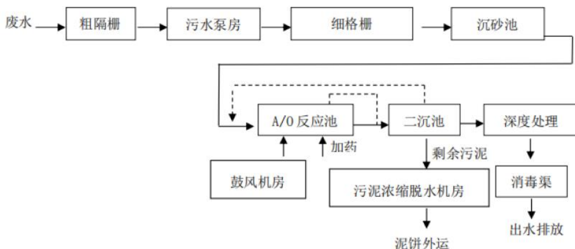
图 3.3-2 导墅污水处理厂污水处理工艺流程
