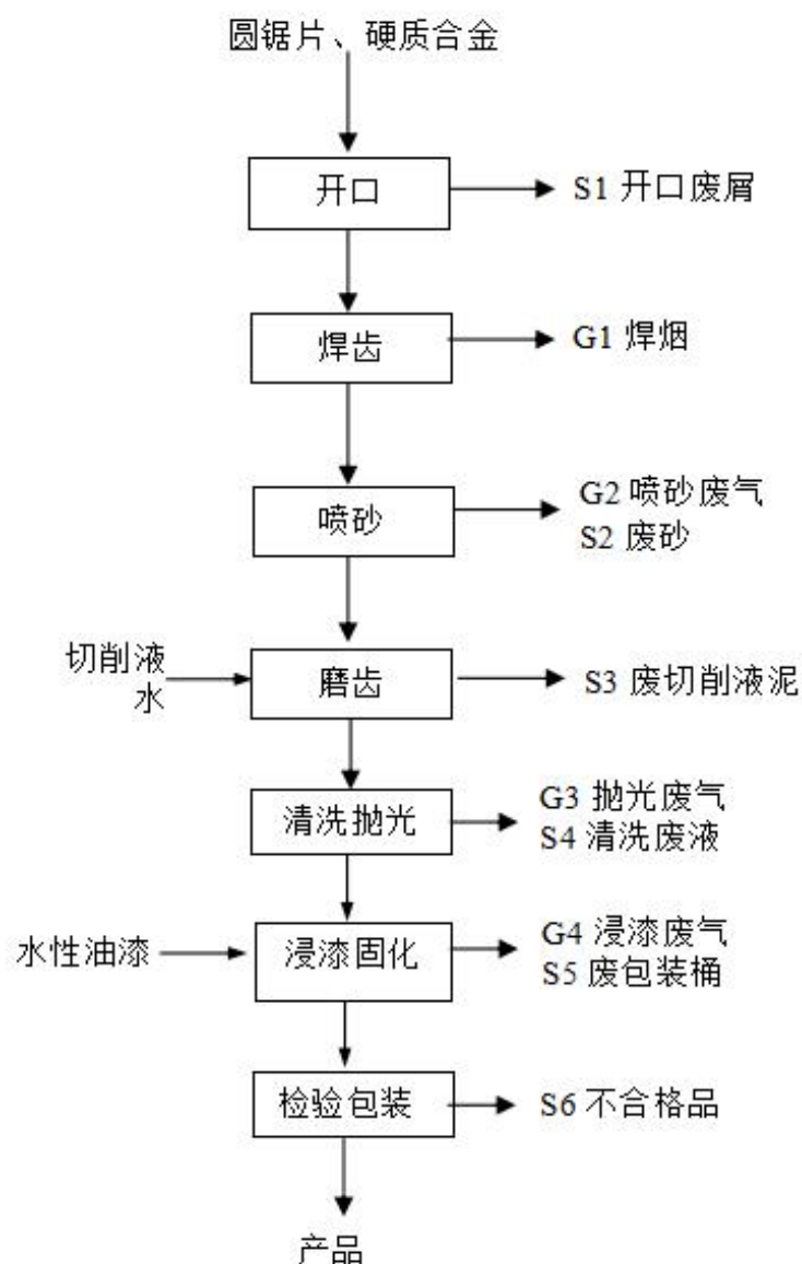
工艺流程及产污环节图
